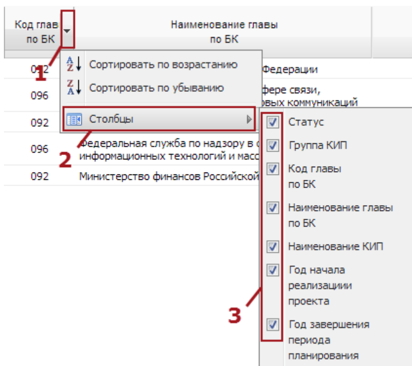
Рисунок 6. Сортировка списка
