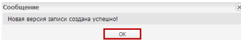
Рисунок 48. Системное сообщение
