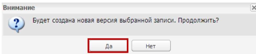
Рисунок 46. Подтверждение действия
