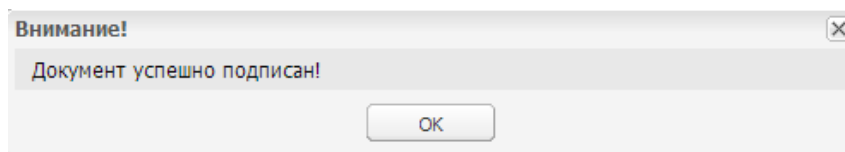
Рисунок 34. Системное сообщение
