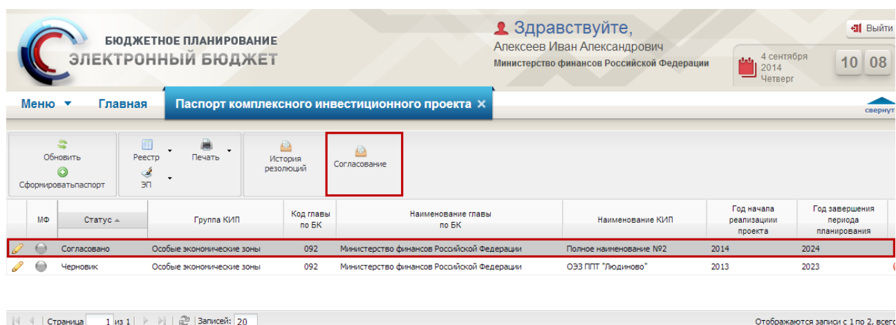
Рисунок 36. Кнопка «Согласование»
